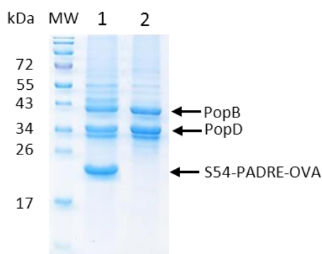
Figure 20: Profil de sécrétion de la souche CHA-OST \Delta uvrA pEAI3S54-PADRE-OVA. Analyse des surnageants de culture par SDS-PAGE. 1. CHA-OST \Delta uvrA pEAI3S54-PADRE-OVA. 2. CHA-OST \Delta uvrA , contrôle négatif. PopB et PopD sont sécrétées dans le milieu, de la même manière que les protéines couplées à ExoS54, lors de l'activation artificielle du SSTT par déplétion calcique.
