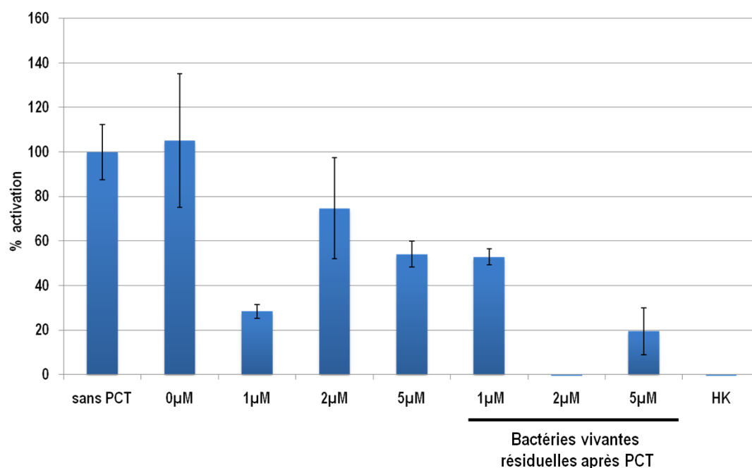
Figure 24 : Présentation par le CMH I d'un peptide issu de l'ovalbumine par les BMDC ayant interagi avec la souche CHA-OST KBMA PEAI3S54-PADRE-OVA exposée à différents PCT (différentes concentrations d'amotosalène). Les barres d'erreur correspondent à la déviation standard (SD). Le graphe représente les résultats d'une seule expérience en triplicat. HK : heat-killed
