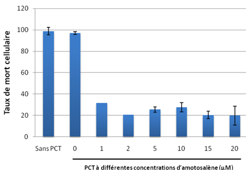
Figure 23 : Mortalité des macrophages J774 après 3h de contact avec la souche CHA-OST \Delta uvrA pEAI3S54-PADRE-OVA (MOI 5:1) traitée ou non par PCT. L'expérience a été réalisée 1 fois en triplicat. Les barres d'erreur correspondent à la déviation standard.
